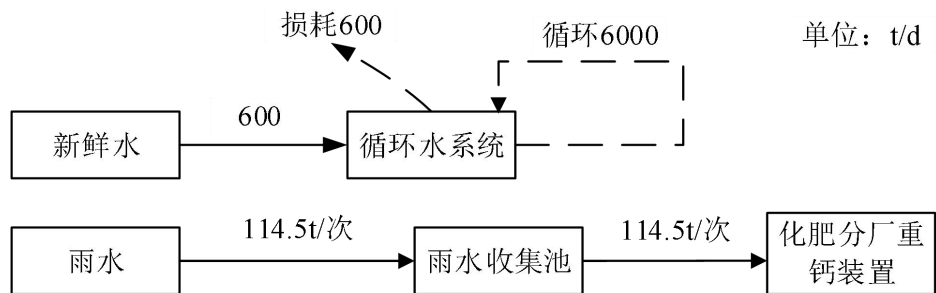
图 5.1-2 扩建项目水平衡图
