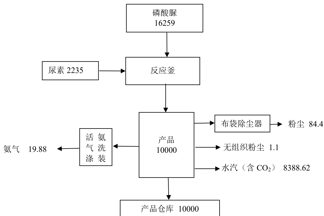
图 5.1-4 物料平衡图 单位: t/a
