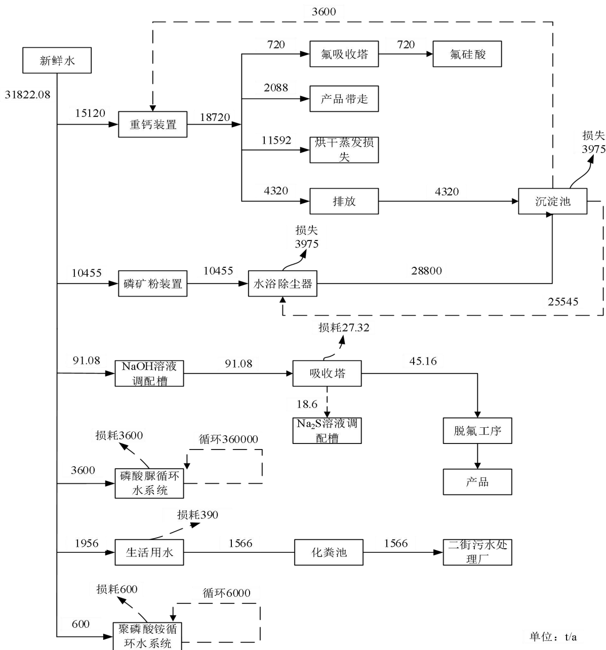
图 5.1-3 扩建后全厂水平衡图（磷酸停产）
