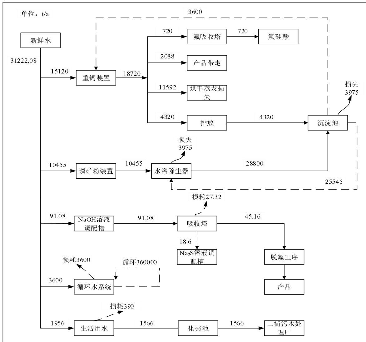
图 3.8-2 现有工程水平衡图（磷酸不生产）
