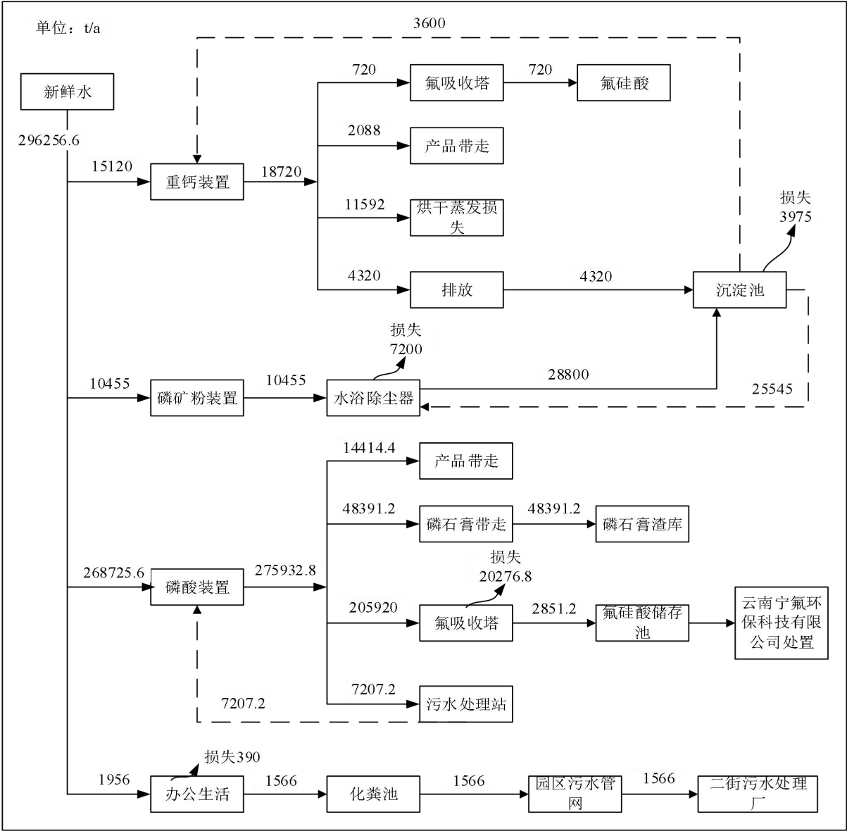
图 3.8-1 现有工程水平衡图（磷酸生产）
